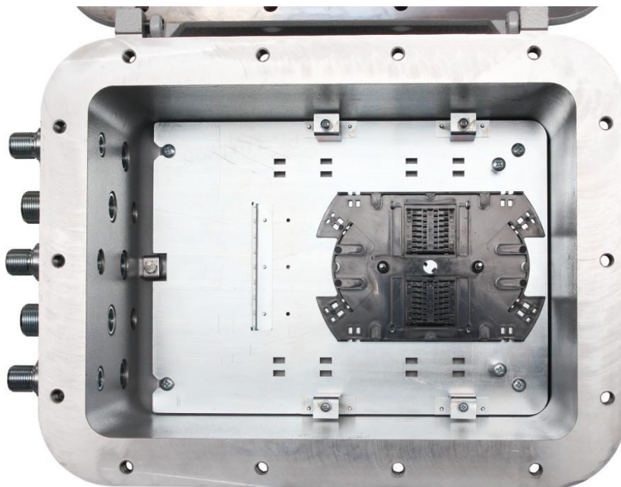
Рисунок 2.4 - Оптический кросс
