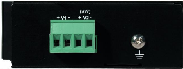
Рис.2 Инжектор Midspan-1/603AG, вид спереди/сбоку
