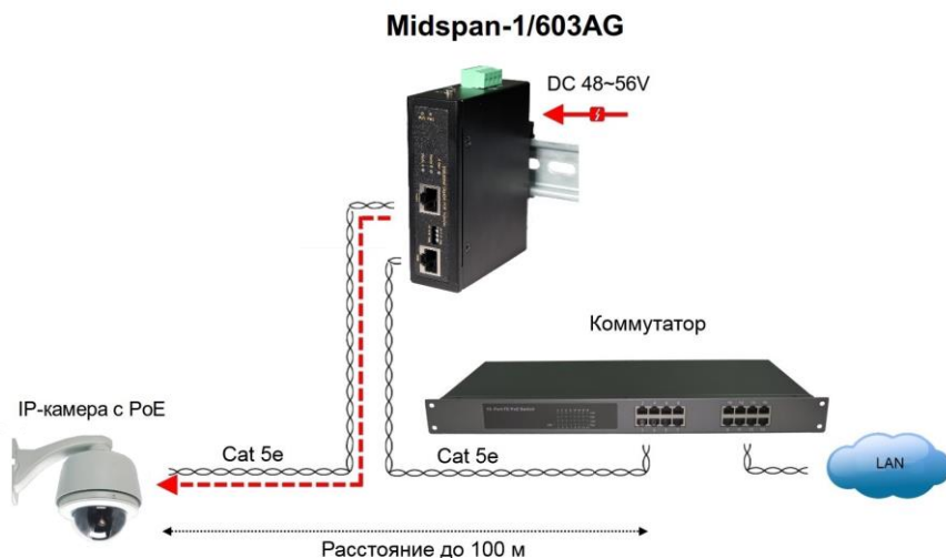
Рис.4 Типовая схема подключения инжектора Midspan-1/603AG
